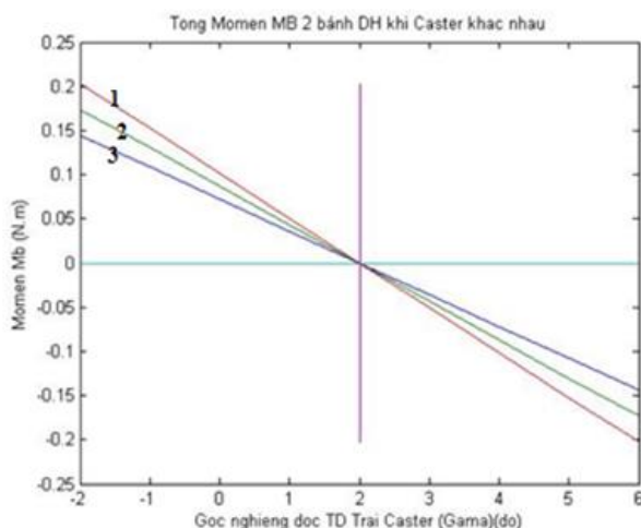
Hình 5: Tổng mô men \sum M_b khi góc Caster trục đứng trái thay đổi 1- Khi xe đầy tải; 2- Khi xe nửa tải; 3- Khi xe không tải
