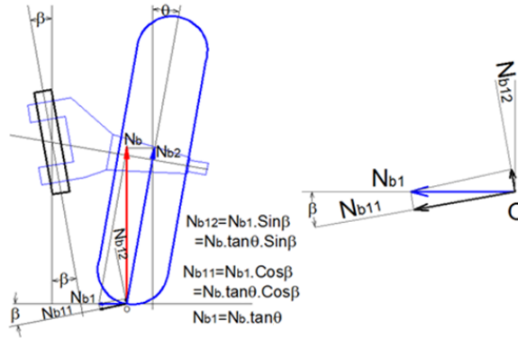
Hình 2: Phản lực tựa N_b có thành phần vuông góc trục đứng N_{b11}
