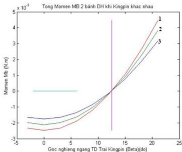
Hình 4: Tổng mô men \sum M_b khi góc Kingpin trục đứng trái thay đổi Đường 1- Khi xe đầy tải; Đường 2- Khi xe nửa tải; Đường 3- Khi xe không tải
