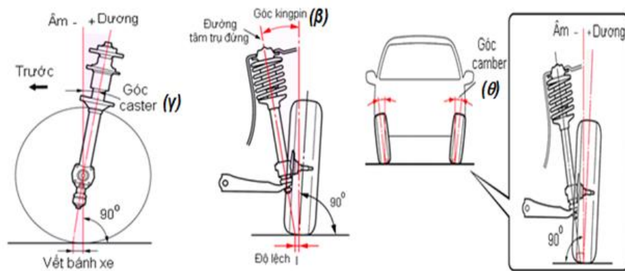
Hình 1: Góc Caster, góc Kingpin và góc Camber
