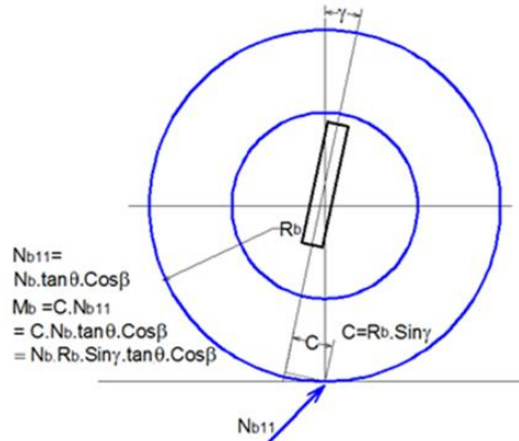
Hình 2: Phản lực tựa N_b có thành phần vuông góc trục đứng N_{b11}
