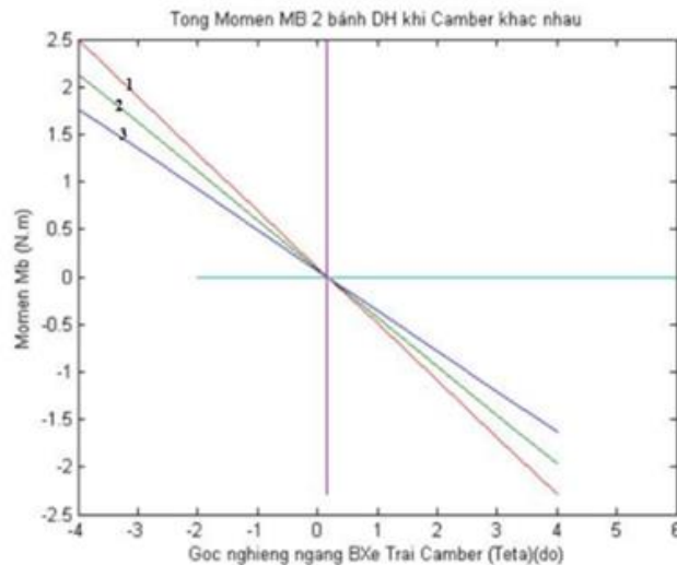
Hình 6: Tổng mô men \sum M_b khi góc Camber bánh xe trái thay đổi Đường 1: Khi xe đầy tải; Đường 2: Khi xe nửa tải; Đường 3: Khi xe không tải
